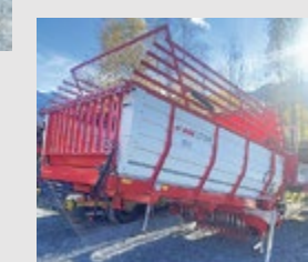
Agrar LD 540 Ausstell-Ladewagen, Jg. 2022, hydr. Rückwand, Picupbreite 1.9 m, Blachrohröffnung, 13 Messer Preis: Fr. 42'000.–
