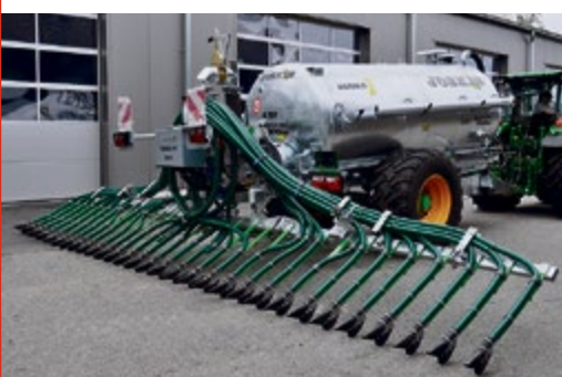
Joskin MODULO 7000 Schleppschuhverteiler 7.5 m Rampe à patin 7.5 m
